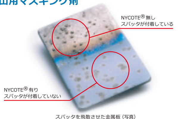
スパッタを飛散させた金属板 (写真)
