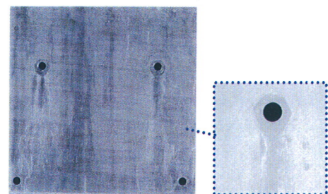
ジオメット®720処理SUSボルト&ナット組付け 拡大写真
